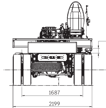
Tampak Belakang
