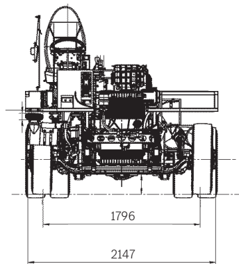
Tampak Depan
